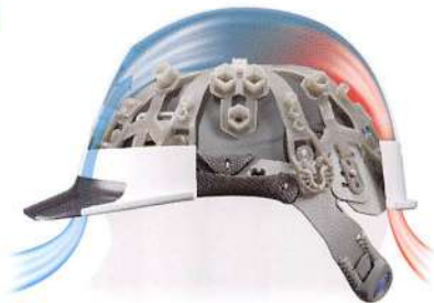
エアライト搭載品の 空気の流れ
